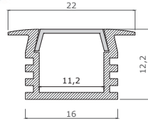
Montageprofil „MAXI-AB“, eloxiert L: 2000mm ART.NR: 111361
