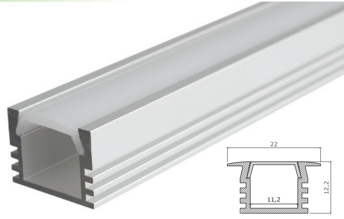
Montageprofil „MAXI-AB“, eloxiert L: 2000mm ART.NR: 111361
