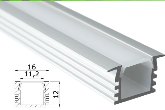
Einbauprofil „MAXI-EB“, eloxiert L: 2000mm ART.NR: 111362
