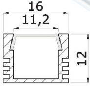
Einbauprofil „MAXI-EB“, eloxiert L: 2000mm ART.NR: 111362
